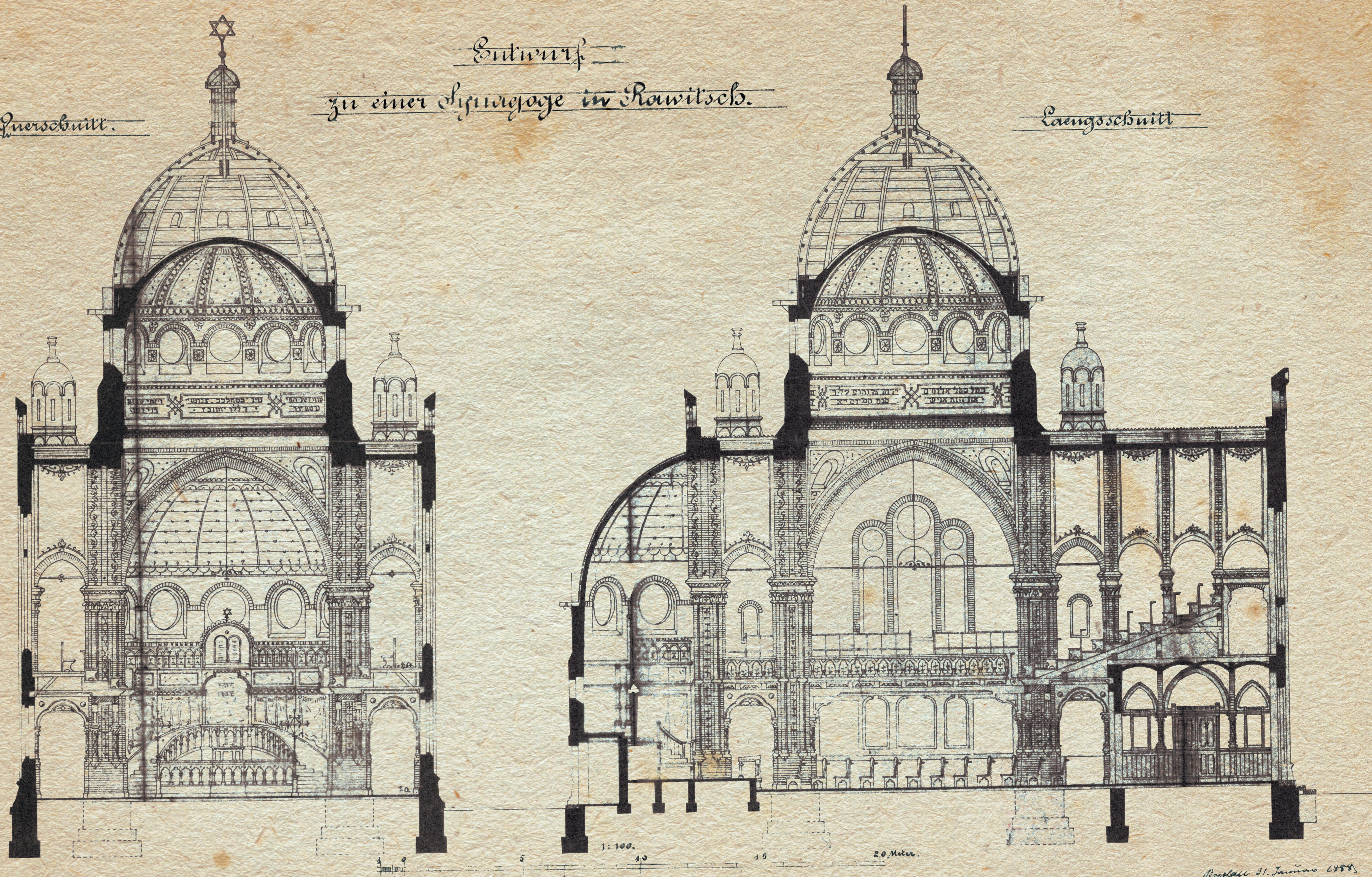
Plan synagogi w Rawiczu, wykonany przez Georga Boettgera (Böttgera), przekrój, 31.01.1888 r.
