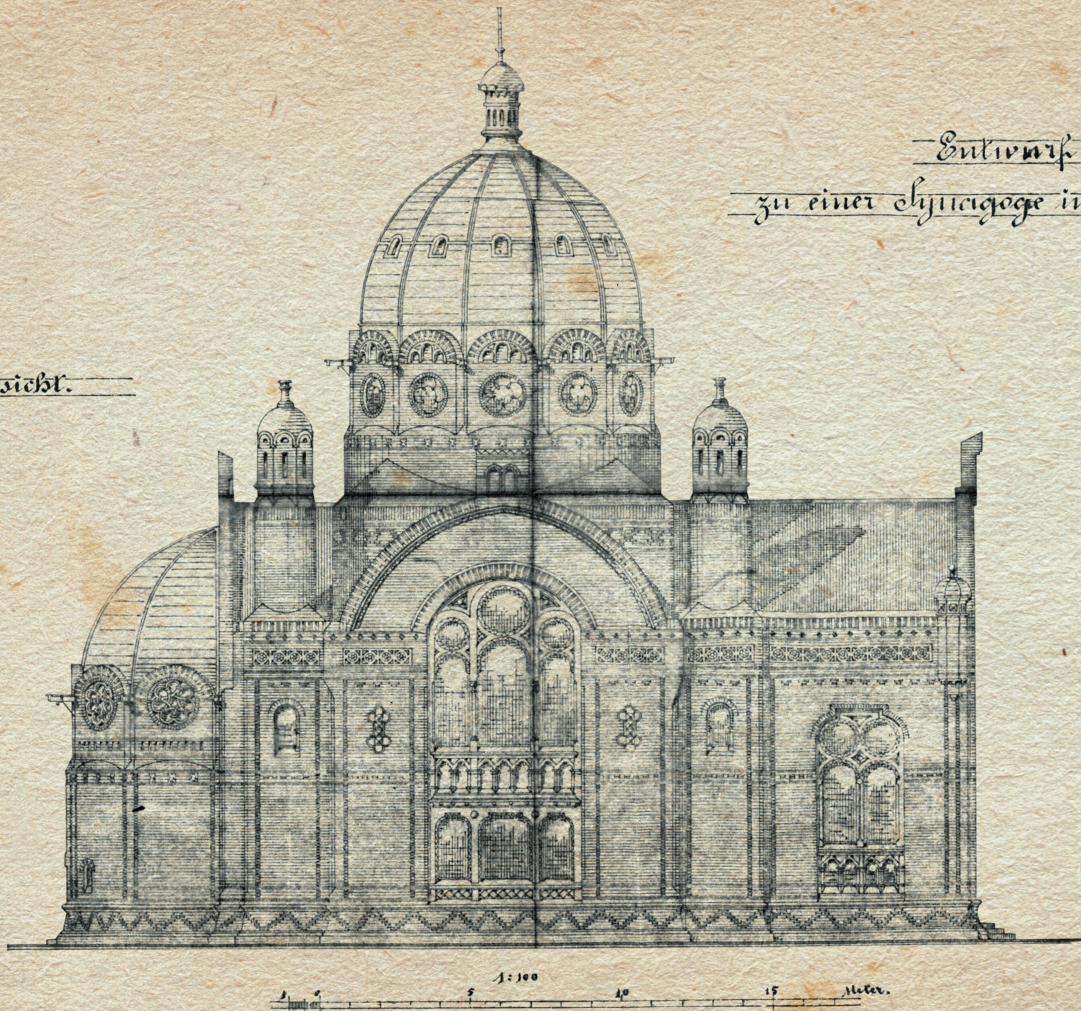
Plan synagogi w Rawiczu, wykonany przez Georga Boettgera (Böttgera), widok południowy, 31.01.1888 r.
